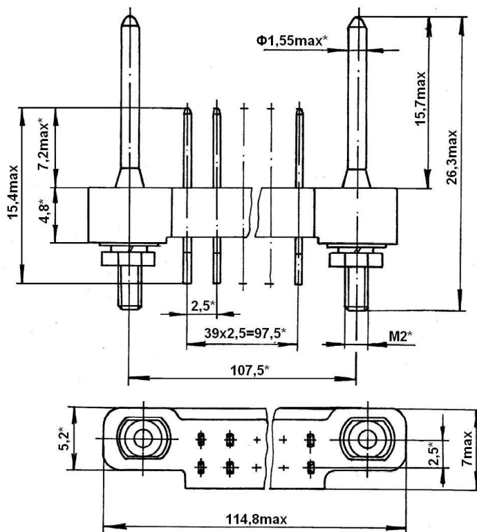
Вилка СНП232-80ВП11-1
