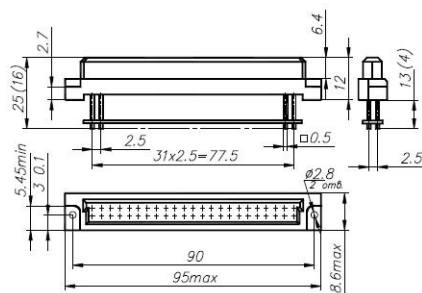
Розетка СНП58
