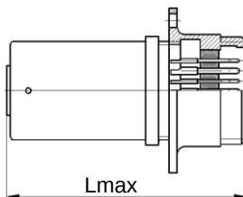
Эскиз - Вилка с кожухом
