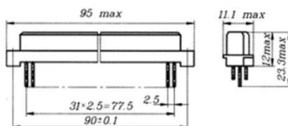
Розетка СНО64
