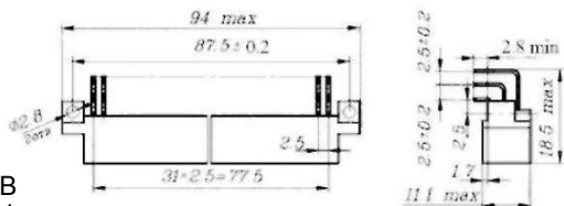
Вилка СНП59
