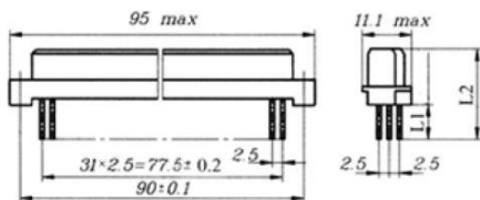
Розетка СНП59
