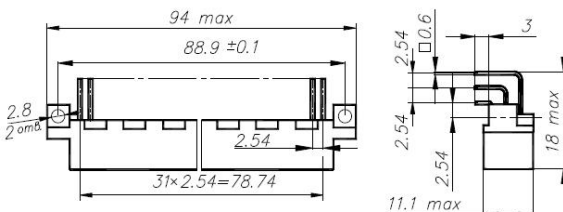
Вилка СНП322
