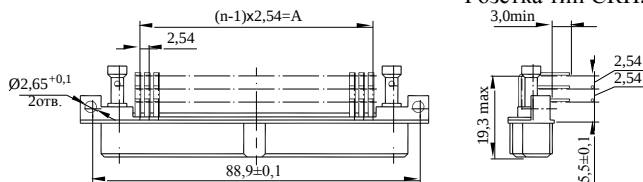
Розетка тип СКП201
