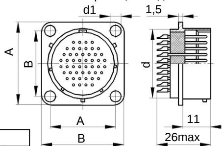
СНЦ31 вилка с фланцем под винты
