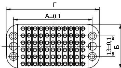
Розетка РПМ12-66Г-Л-В
