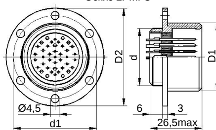
Эскиз 2РМГСД
