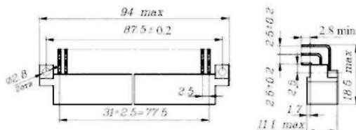
Вилка СНП59
