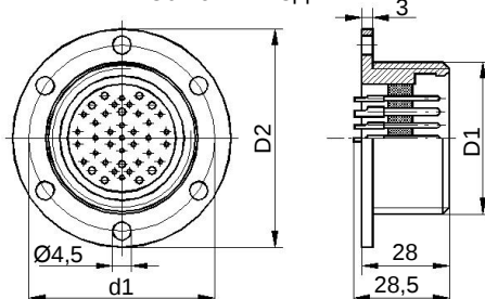
Эскиз 2РМГСД
