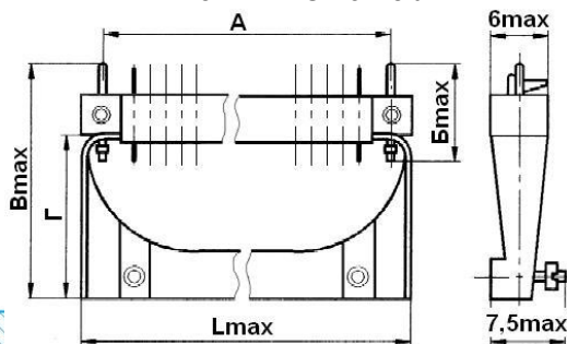
Вилка РПМ13-20Ш6-Л-В
