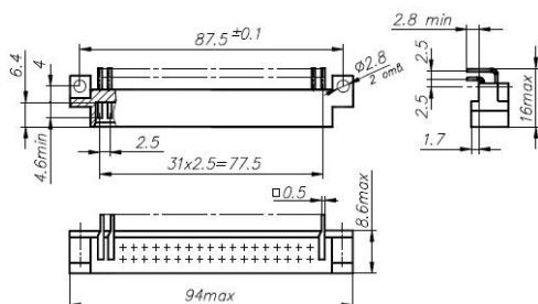
Вилка СНП58
