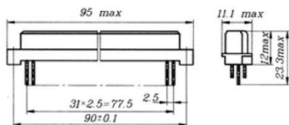
Розетка СНО64
