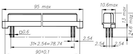
Розетка СНП322
