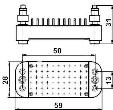
Розетка РПМ12М
