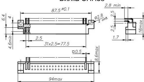
Вилка СНП58
