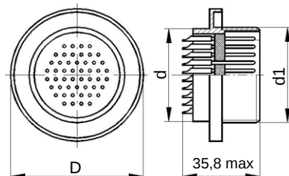
Эскиз – РРМ44
